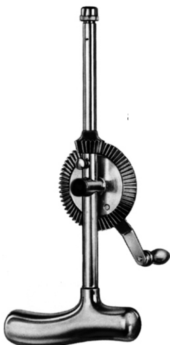
Stille-Sherman 8447.24 24 cm compl. incl. 8447.25 - 8447.35
