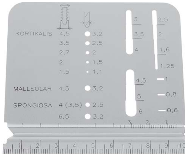
DH-710-00B Messlehre für Schrauben Measuring Plate for screws Medidor para tornillos
