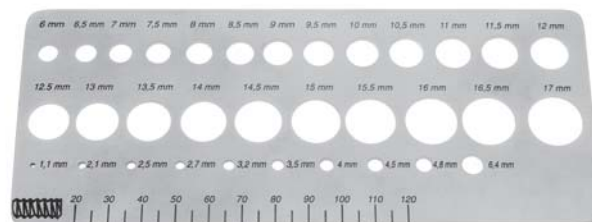
DH-560-00A Lochlehre für Nägel Measuring Gauge for Nails Medidor para Clavos
