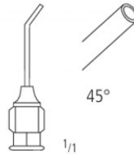
GILLS-WELSH KP 745/25 3,0 cm/1 1/4" 25G
