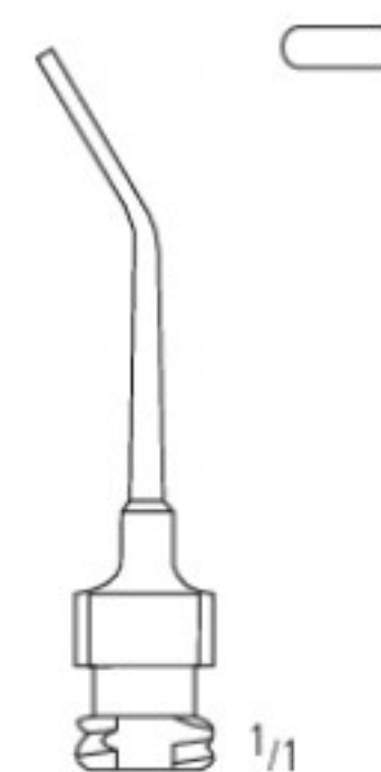
MODELL BONN 4,0 cm/1 1/2" KP 705/19 KP 705/20 19G 20G
