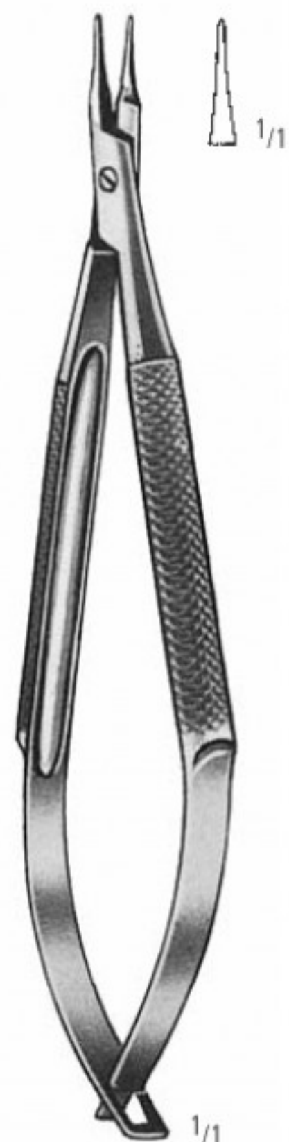
BARRAQUER- TROUTMAN AE 602/10 10,0 cm/4"
